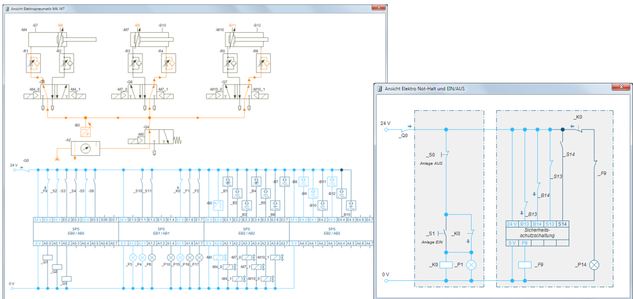
Elektropneumatische Schaltung für die Zylinder
